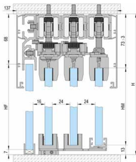
Montage plafond / 3 vantaux / avec pan fixe
