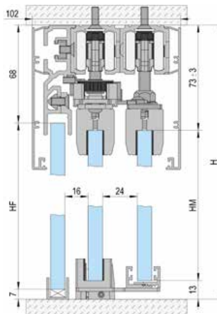
Montage plafond / 2 vantaux / avec pan fixe
