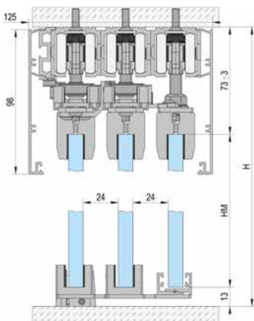
Montage plafond / 3 vantaux
