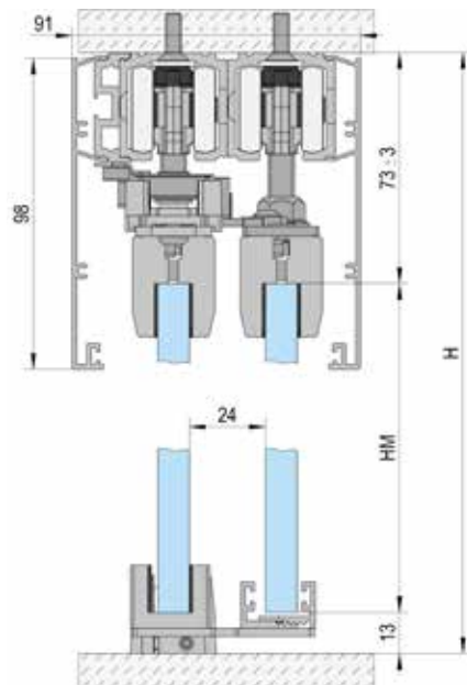
Montage plafond / 2 vantaux
