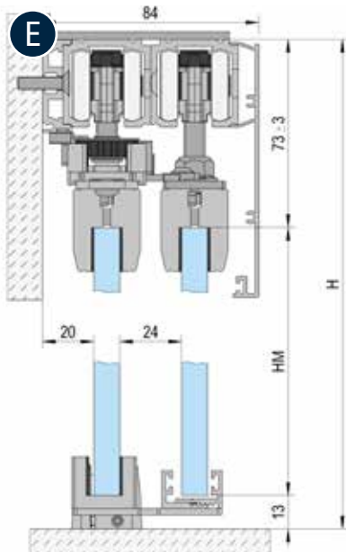
Montage mural / 2 vantaux
