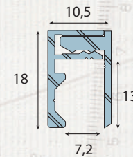
R 702 U égal à clip
