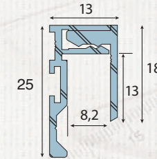
R 802 U inégal à clip
