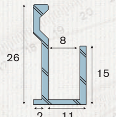
R 900 U inégal
